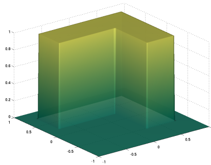
(b) target y_{d,2}
